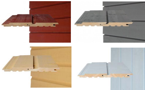
Puu-ulkoverhoukset toimitetaan valmiiksi tilattuun väriin maalattuna. Paneelien päätkin on pontattu ja kiinnitystapa on piilonaulaus. Näin saadaan pintavalmista, naulanreiätöntä seinää ympäri vuoden.
